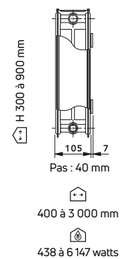
MODÈLE 22KV Sans étriers
