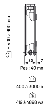
MODÈLE 21KV Sans étriers
