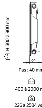
MODÈLE 11KV Avec étriers
