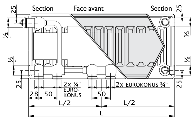
Radiateur avec vanne à gauche (rad retourné)
