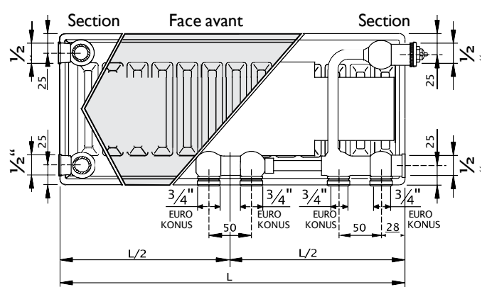
Radiateur avec vanne à droite
